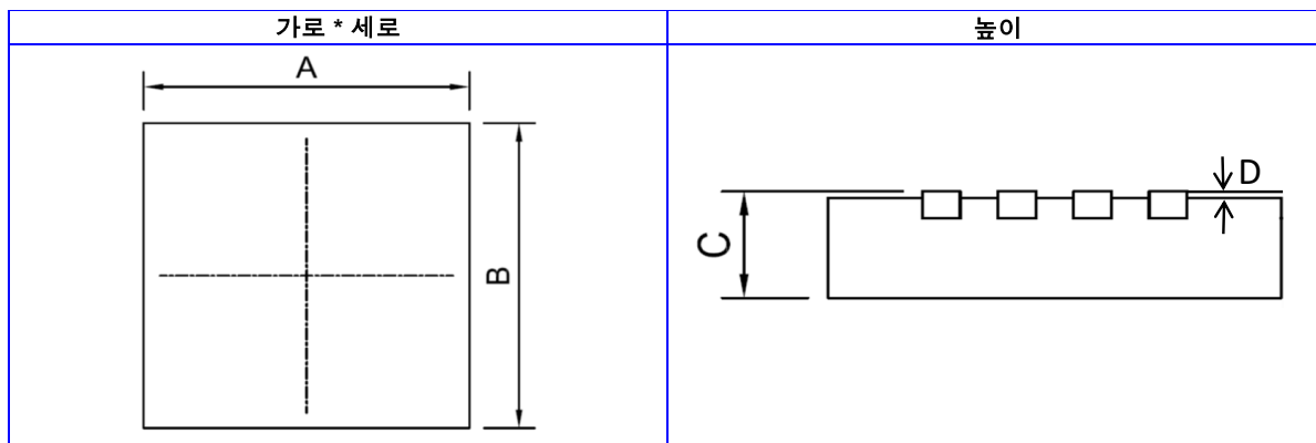
■ Actual PKG Dimension Data
